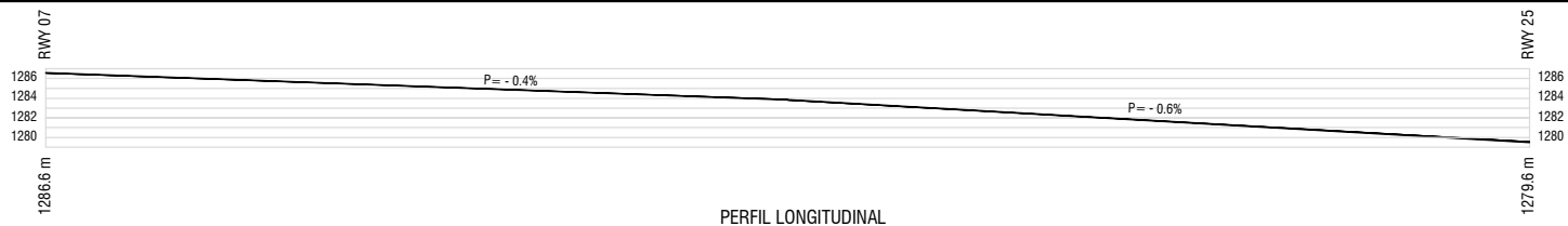
PERFIL LONGITUDINAL
