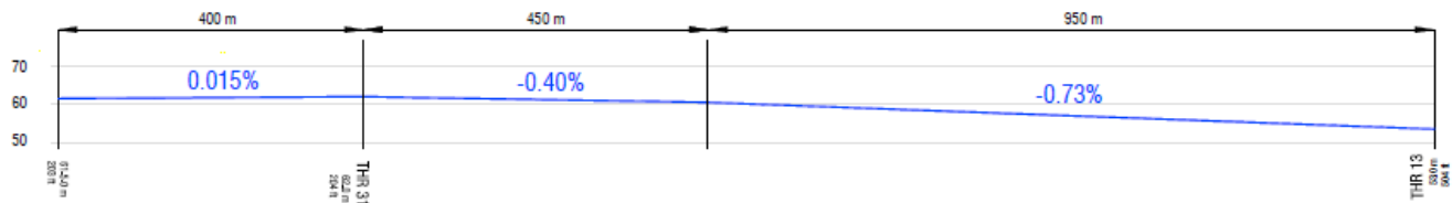
PERFIL LONGITUDINAL PISTA
