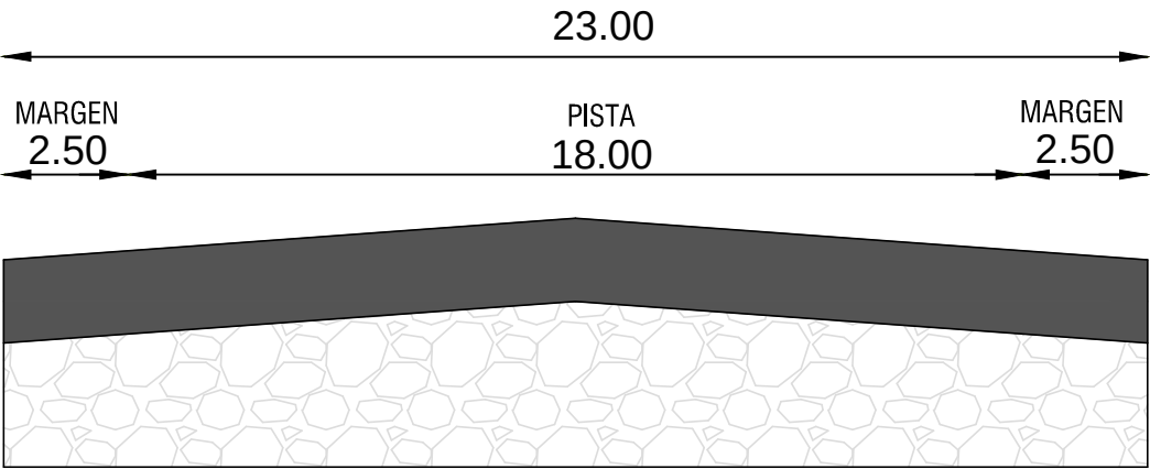
PERFIL TRANSVERSAL
